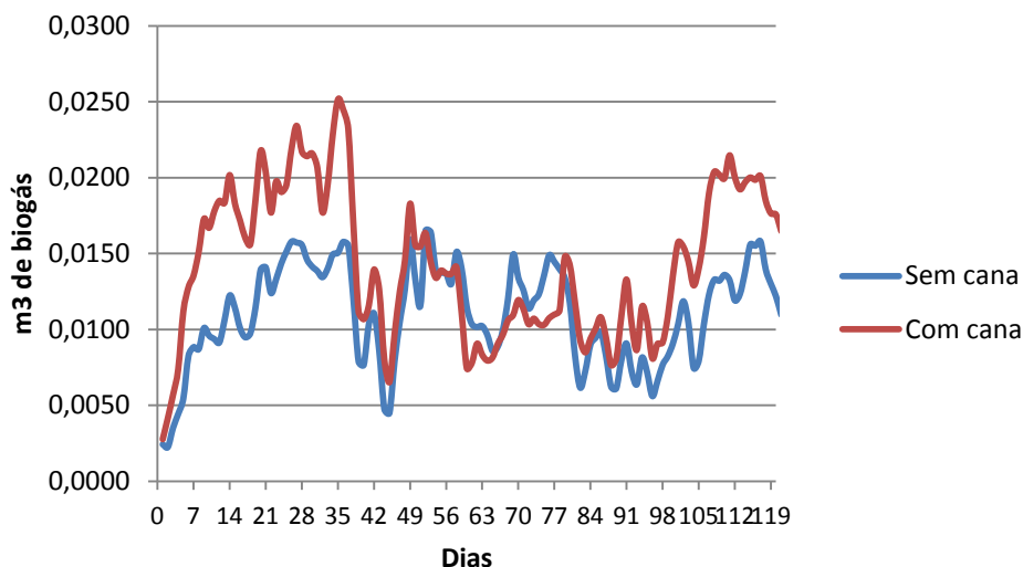
Figura 1. Distribuição da produção diária de biogás (m 3 ) ao longo do período experimental
